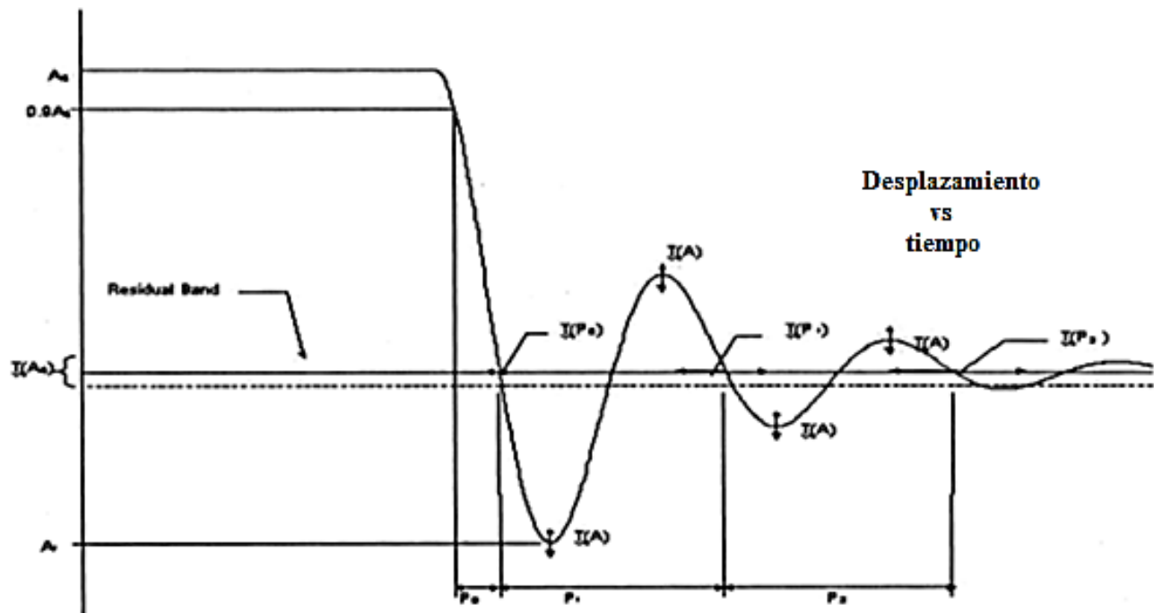
Figura 3.2A Respuesta al movimiento momentáneo de un sistema de baja amortiguación.
